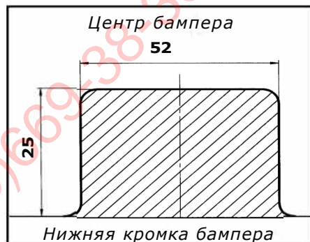
СХЕМА ВЫРЕЗА
